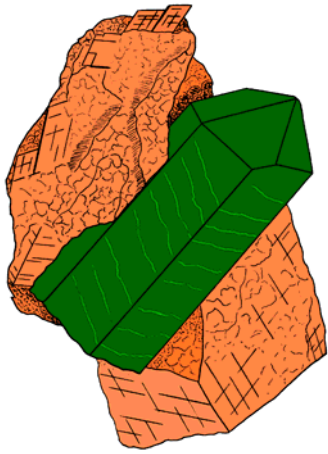
Apatite
