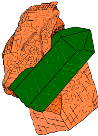
Apatite
