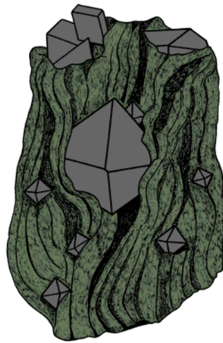
Magnetite
