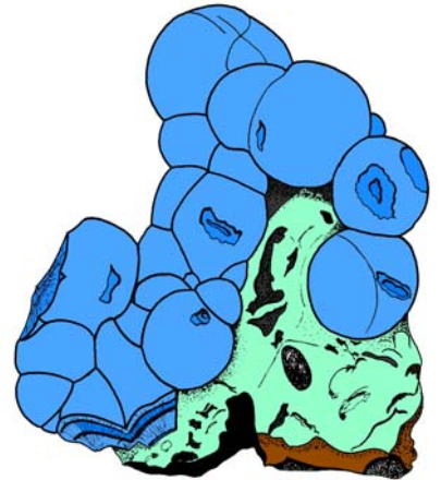
Azurite
