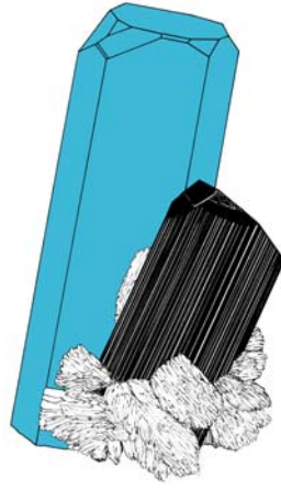
Aquamarine
