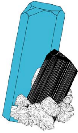
Aquamarine
