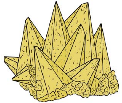
Calcite
