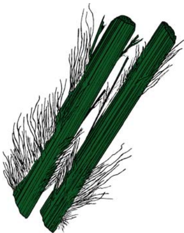
Asbestos
