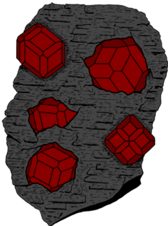
Garnet
