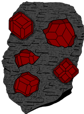
Garnet
