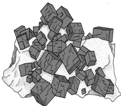
Galena
