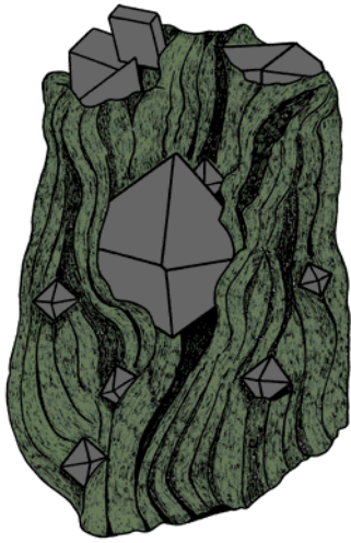
Magnetite
