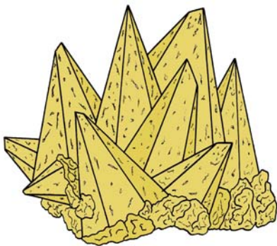
Calcite
