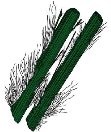
Asbestos
